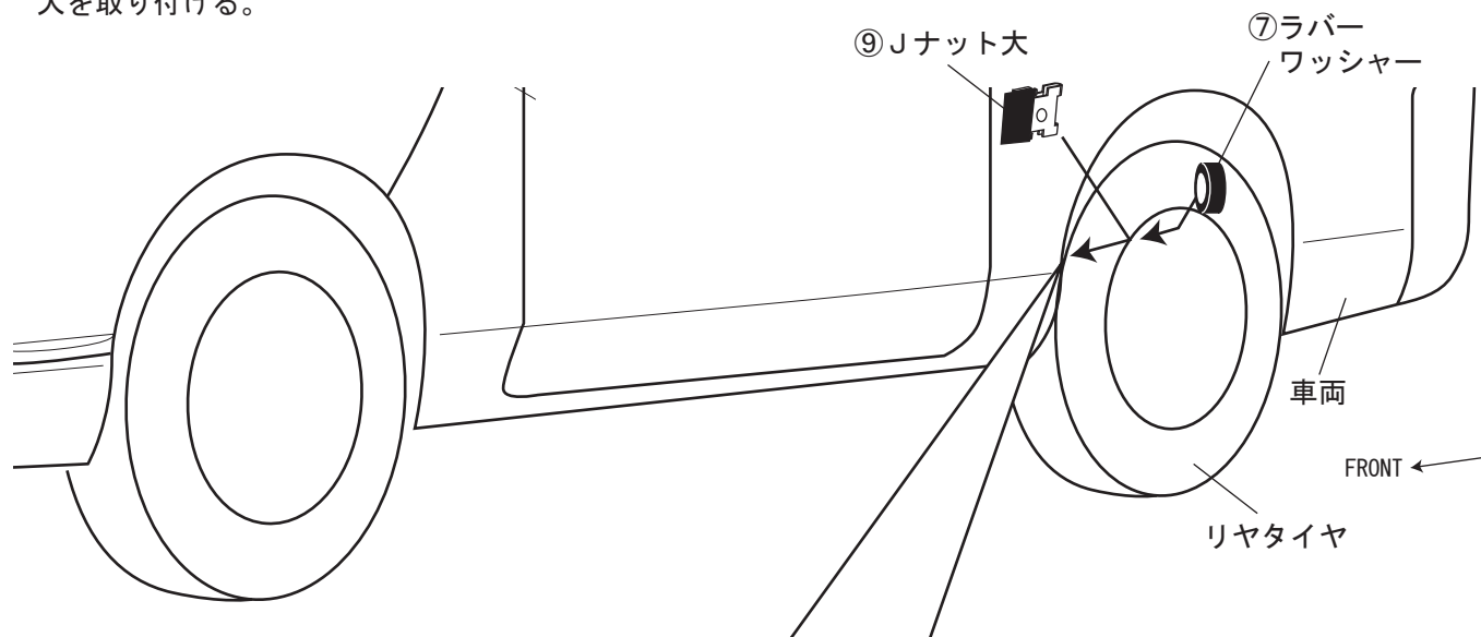
⑦ラバーワッシャー ⑨Jナット大 取り付け詳細図
