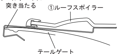
[A-A 断面図]
