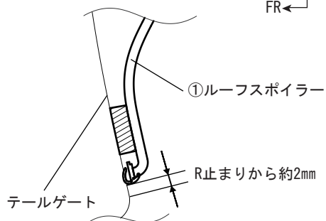
[B-B 断面図]
