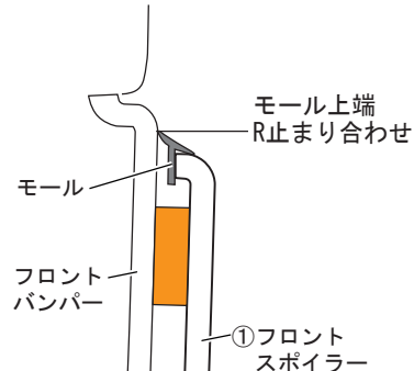
D-D断面図
