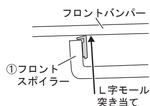
B-B断面図
