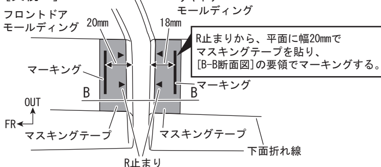
[矢視 b]
