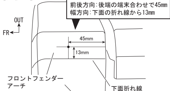
[矢視 a]
